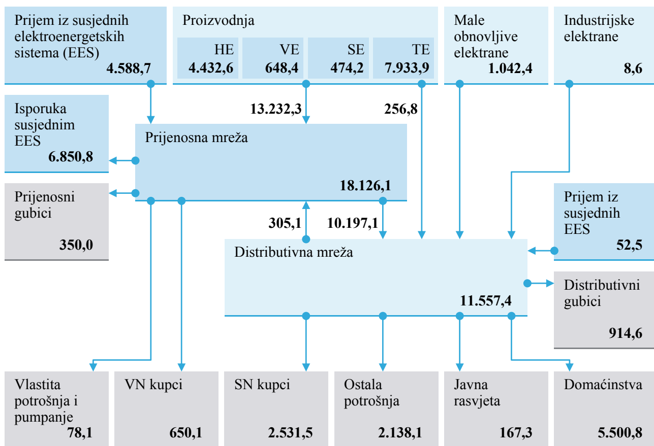
Slika 9. Ostvarene bilansne veličine u 2025. godini (GWh)
