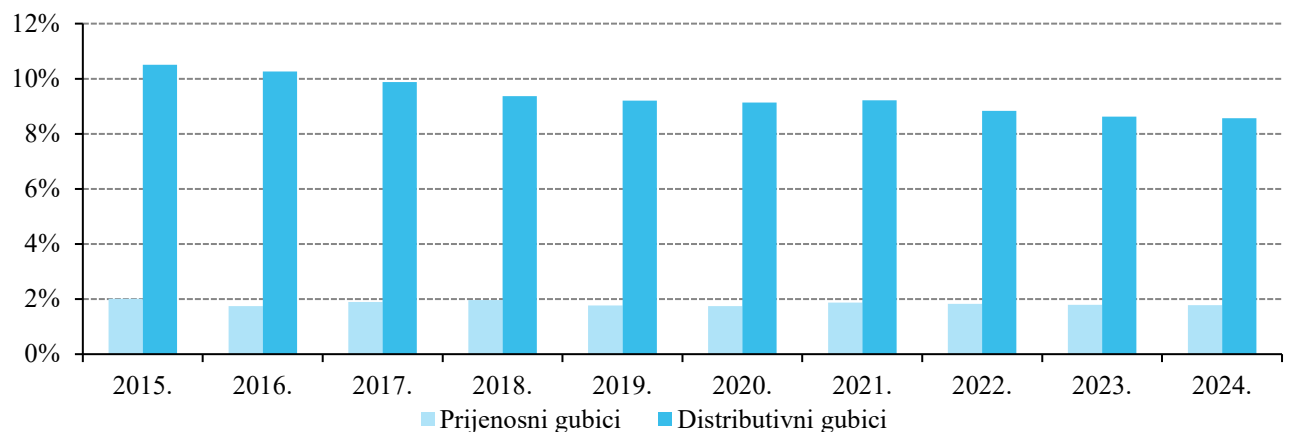
Slika 4. Prijenosni i distributivni gubici
